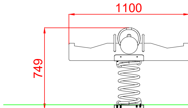
ALZADO
