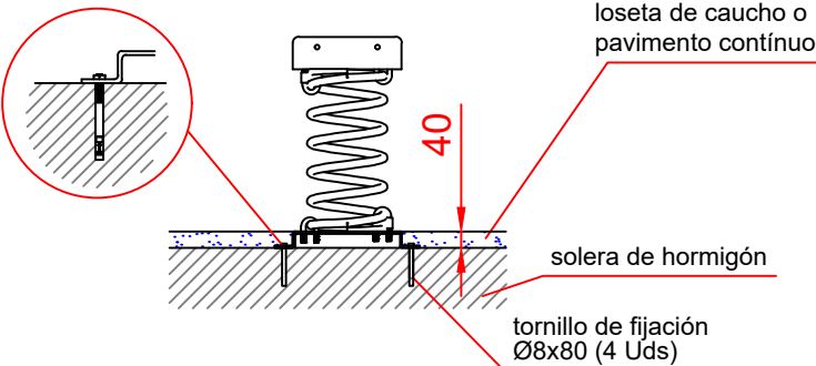
Detalle de sujeción de espiral metálica
