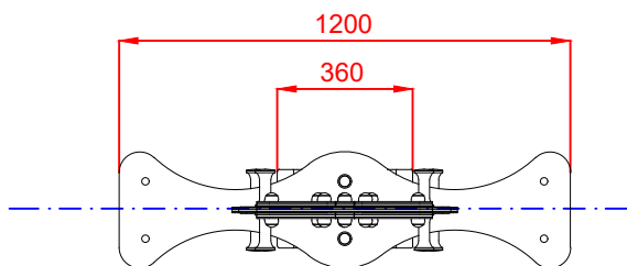
PLANTA
