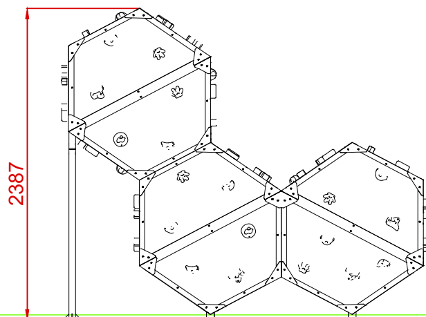
ALZADO
