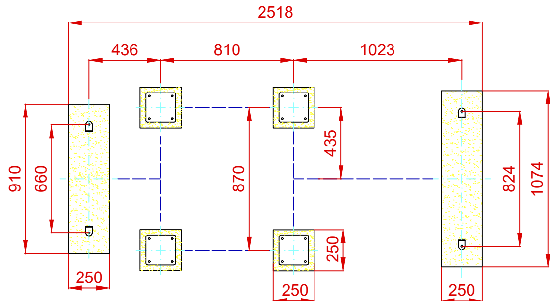
PLANTA CIMENTACIÓN
