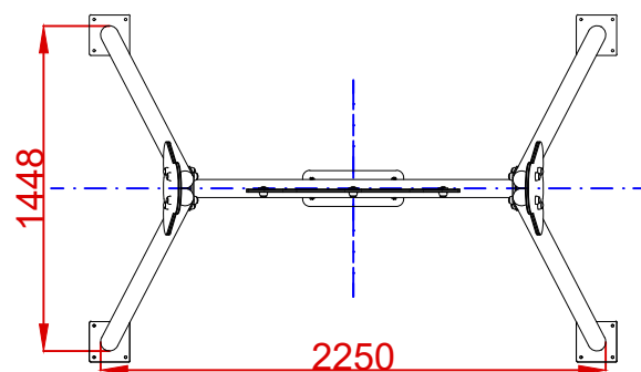
PLANTA
