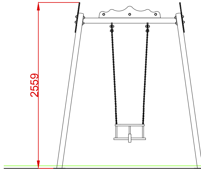
ALZADO
