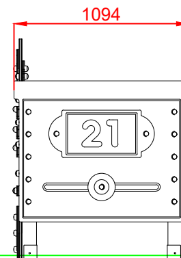
PERFIL IZQUIERDO
